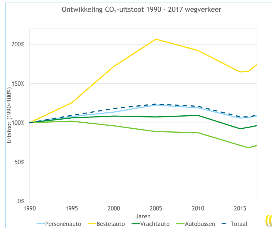
Figuur 4 - Ontwikkeling CO 2 -uitstoot voor wegverkeer per modaliteit
